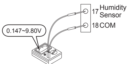
[Abb. 7] Spannung des Feuchtigkeitssensors
