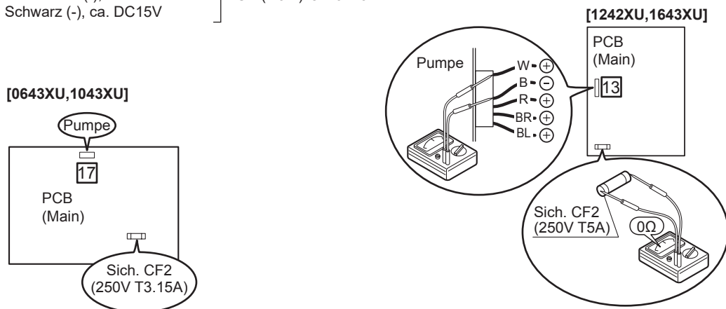
[Abb. 4] Widerstand d. Spule des 4-Wege Ventils
